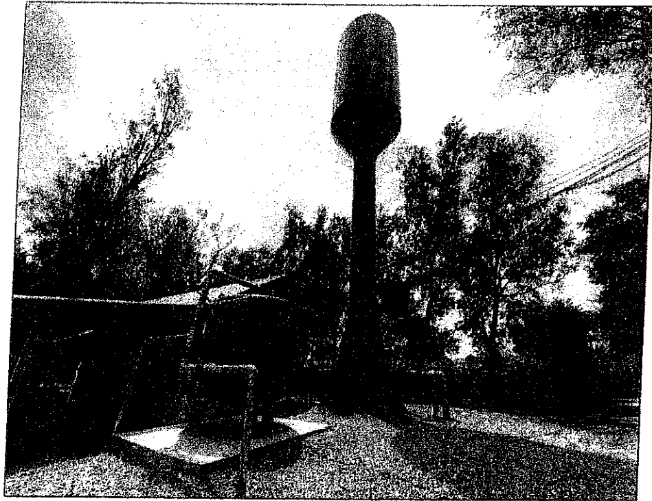
ระบบประปาบาดาลสูบน้ำบาดาลด้วยระบบไฟฟ้าพร้อมจุดจ่ายน้ำดื่มน้ำใช้
